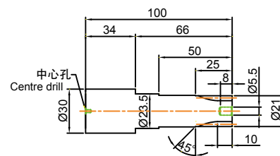
入力軸(B型) 尺寸圖
