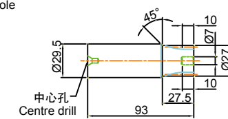
入力軸(A型) 尺寸圖
