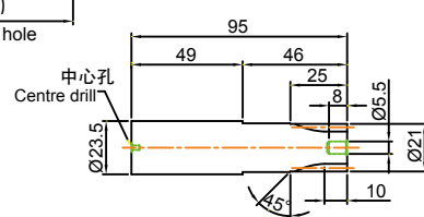
入力軸(A型) 尺寸圖
