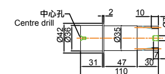
入力軸(A型) 尺寸圖
