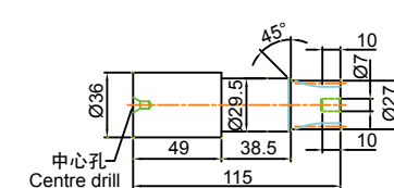
輸入軸(B型) 尺寸圖
