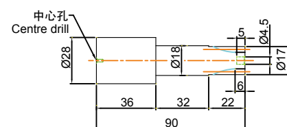
入力軸(A型) 尺寸圖
