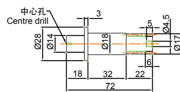
入力軸(B型) 尺寸圖
