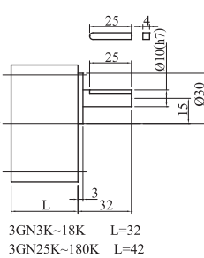
●減速機 3GN3K-180K
