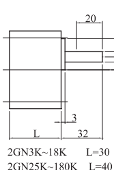
●減速機 2GN3K-180K
