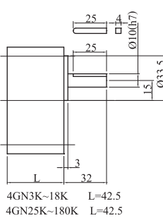
●減速機 4GN3K-180K
