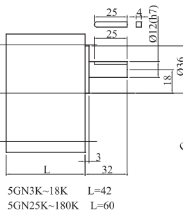
●減速機 5GN3K-180K
