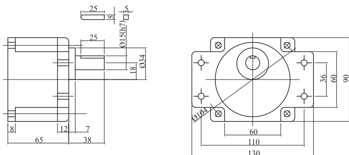
●減速機 5GU3K-180K
