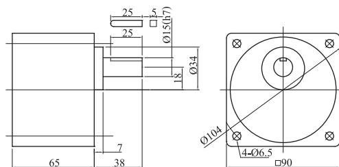
●減速機 5GU3KB-180KB
