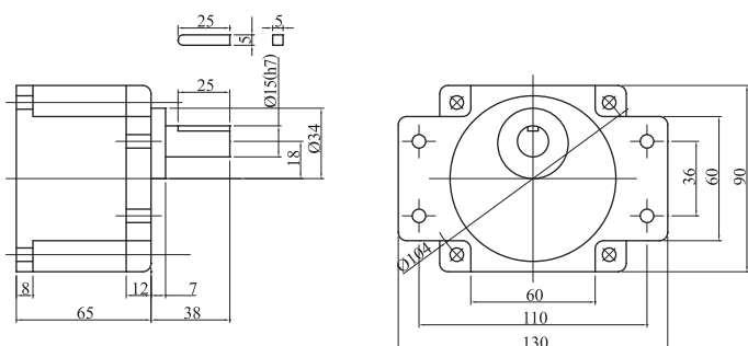
●減速機 5GU3K~180K
