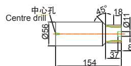
入力軸(A型) 尺寸圖
