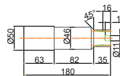
入力軸(B型) 尺寸圖
