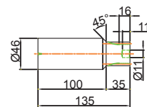
入力軸(A型) 尺寸圖
