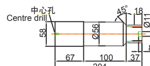
入力軸(B型) 尺寸圖
