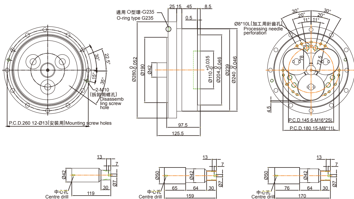
入力軸(A型) 尺寸圖 Input shaft (A type) dimensions
