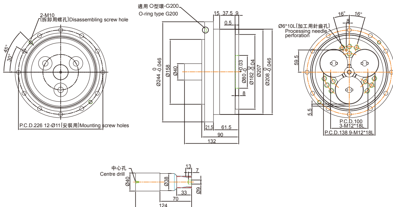
入力軸 尺寸圖 Input shaft dimensions
