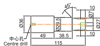
入力軸(B型) 尺寸圖 Input shaft (B type) dimensions
