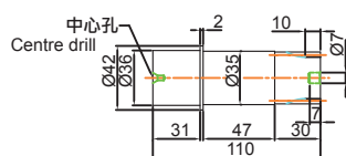
入力軸(A型) 尺寸圖 Input shaft (A type) dimensions
