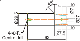
入力軸(A型) 尺寸圖 Input shaft (A type) dimensions
