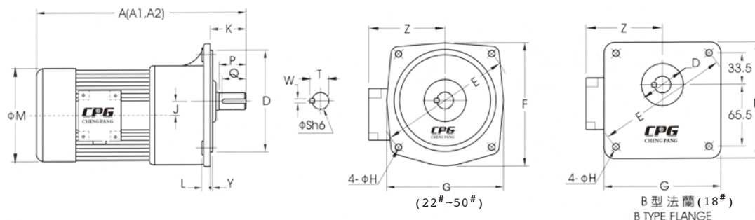
出力軸尺寸 OUTPUT SHAFT
