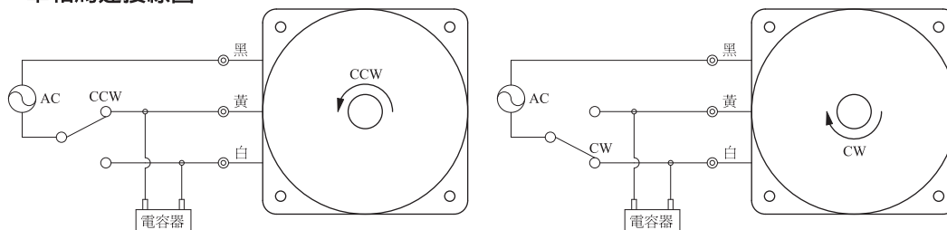
單相馬達接線圖
