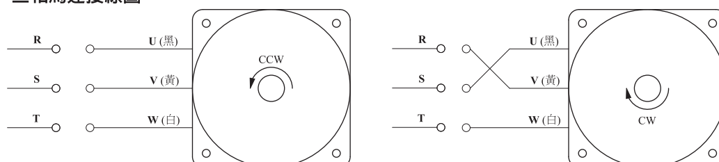
三相馬達接線圖
